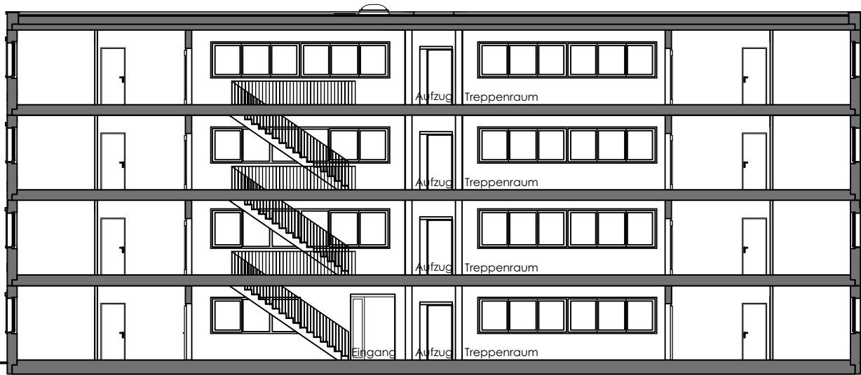
Schnitt A-A
