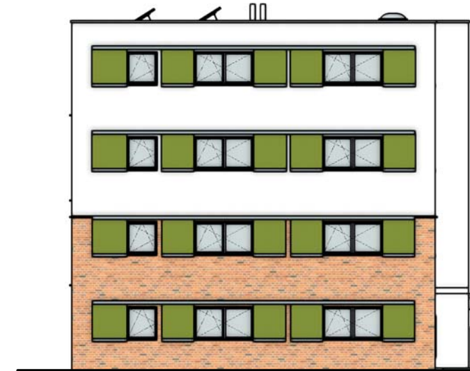
Ansicht West
